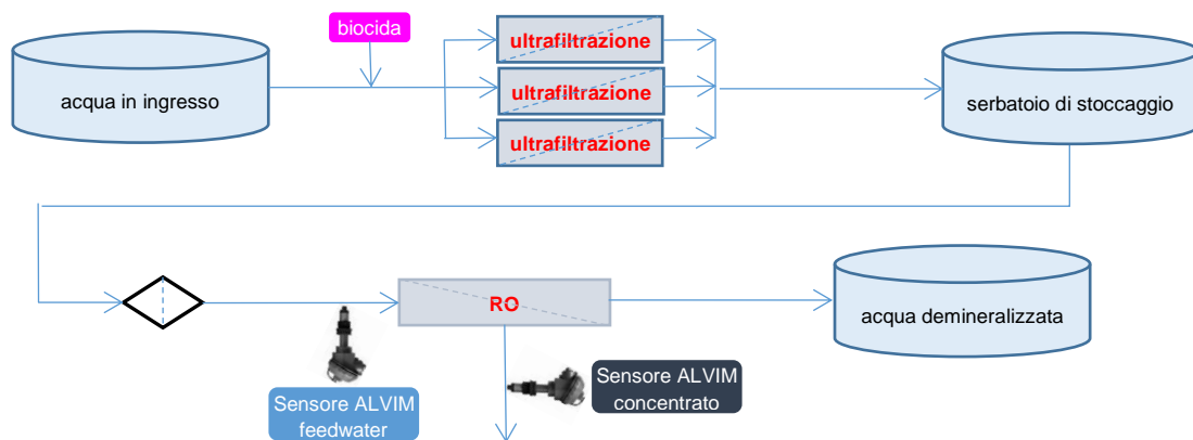
Figura 1: Schema del sistema RO
